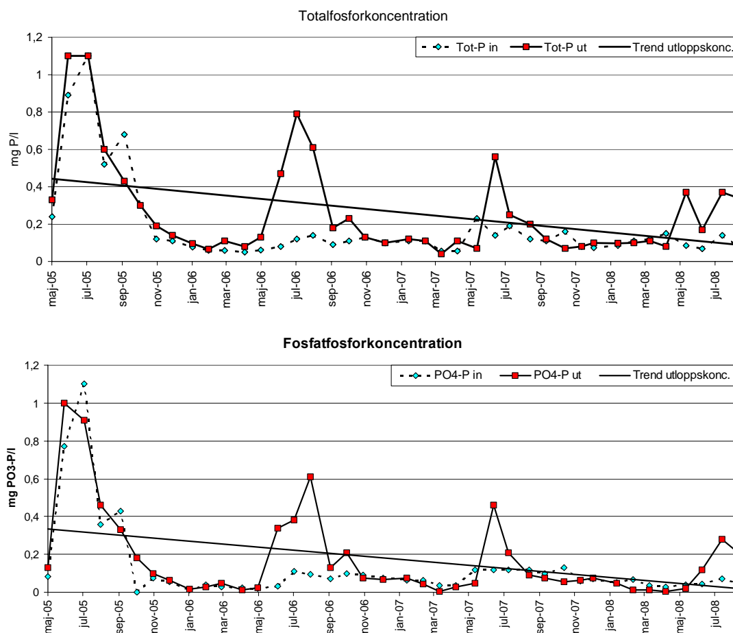
Figur 12. Uppmätta totalfosfor- och fosfatfosforhalter i in- och utlopp från Näsbyholmsjön under 40 mättilfällen mellan maj 2005 och augusti 2008.
