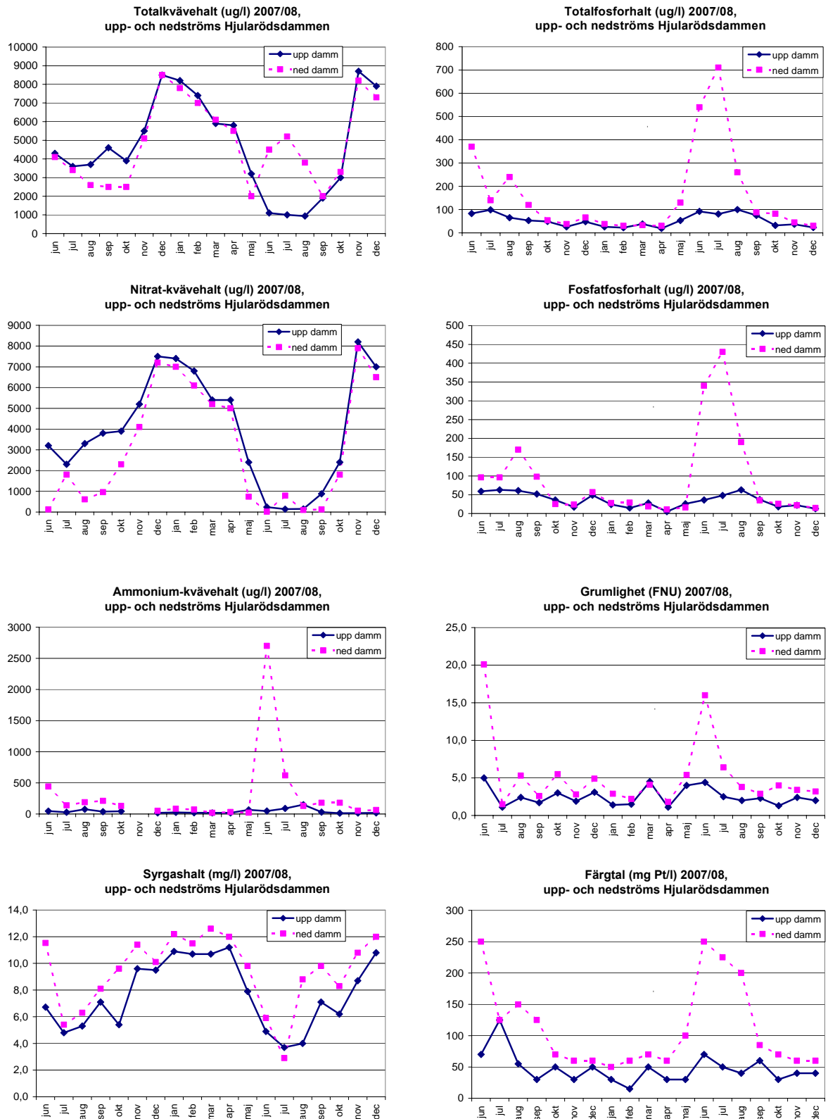
Figur 8. Analysdata från åtta parametrar uppströms och nedströms Hjularödsdammens våtmarker vid 19 mättillfällen under 2007/2008. Värderna under detektionsgränser har satts till 0.
