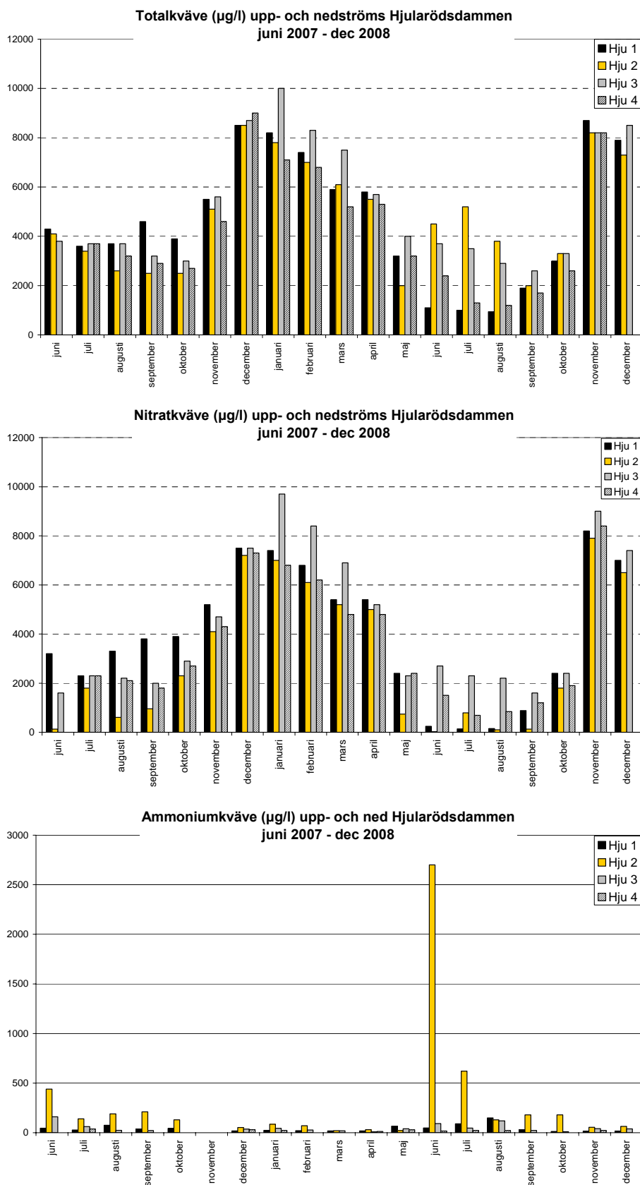
Figur 9. Totalkväve, nitratkväve och ammoniumkväve uppströms (Hju 1) och nedströms (Hju 2, 3 och 4) Hjarlarödsdämmen juni 2007 till december 2008.
