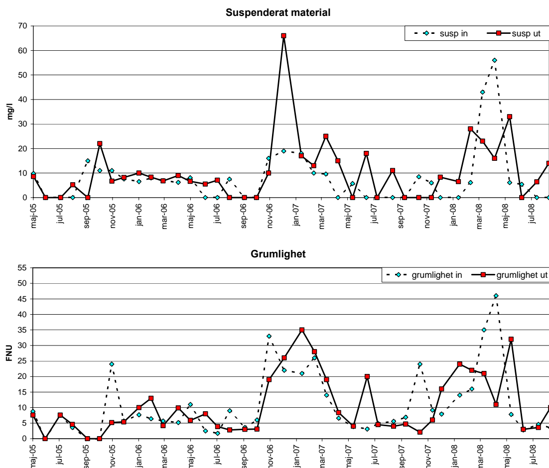
Figur 13. Uppmätt halt suspenderat material samt grumlighet i in- och utlopp från Näsbyholmssjön under 40 måttillfällen mellan maj 2005 och augusti 2008.
