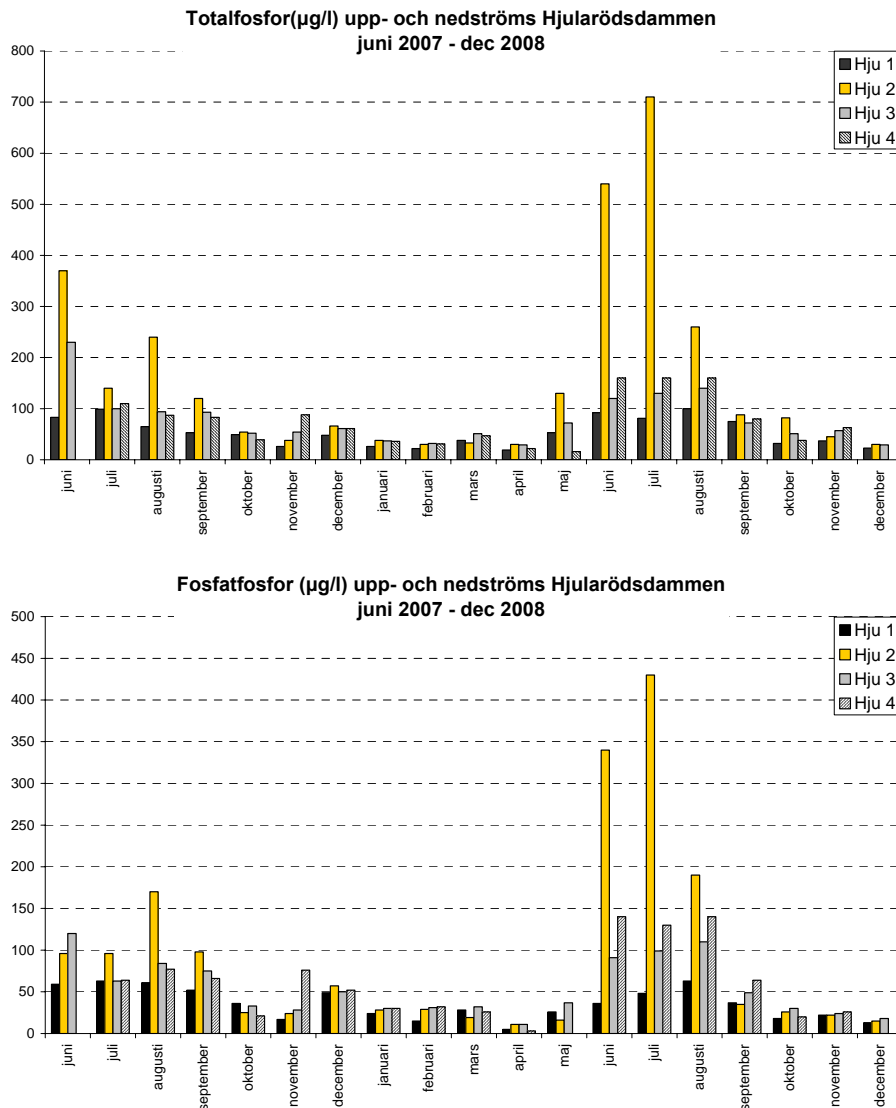
Figur 10. Totalfosfor och fosfatfosfor uppströms (Hju 1) och nedströms (Hju 2, 3 och 4) Hjulärösvåtmarken juni 2007 till december 2008.
