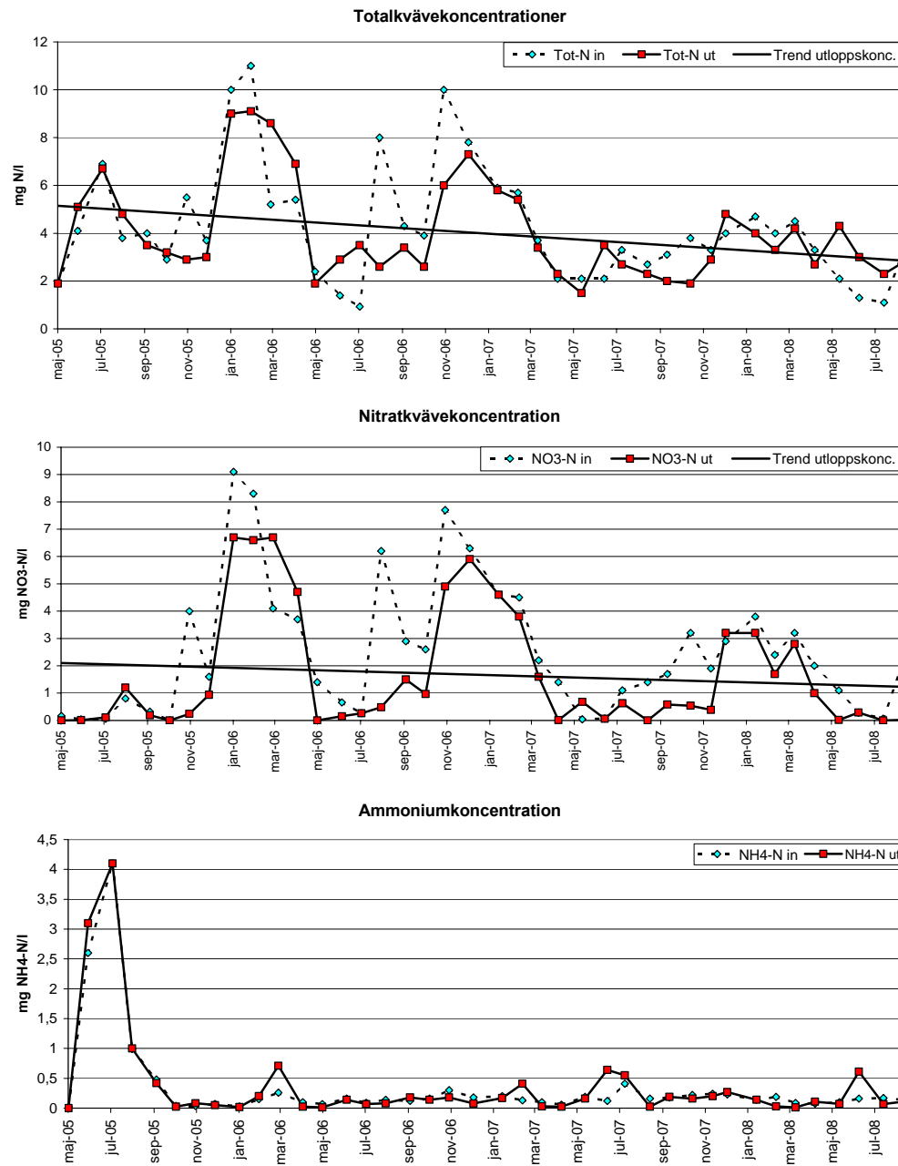
Figur 11. Uppmätta totalkväve-, nitratkväve- och ammoniumkvävehalter i in- och utlopp från Näsbyholmssjön under 40 mätillfällen mellan maj 2005 och augusti 2008.
